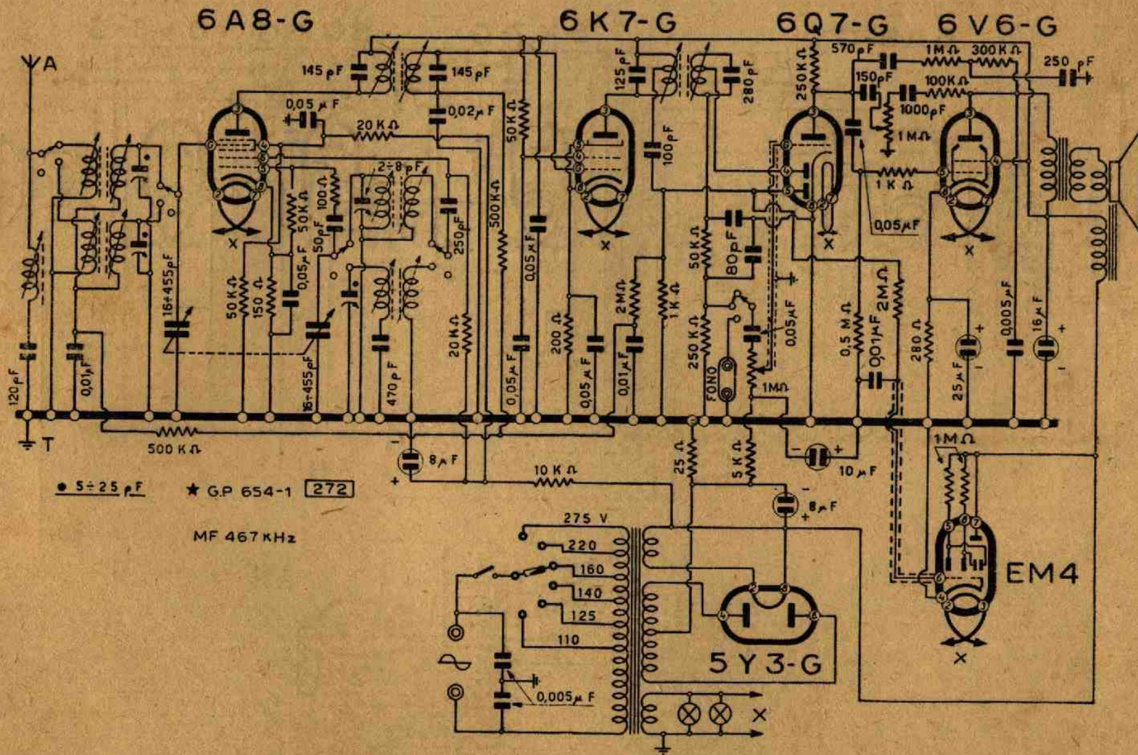
Lo schema elettrico del "C. G. E. 355,."
