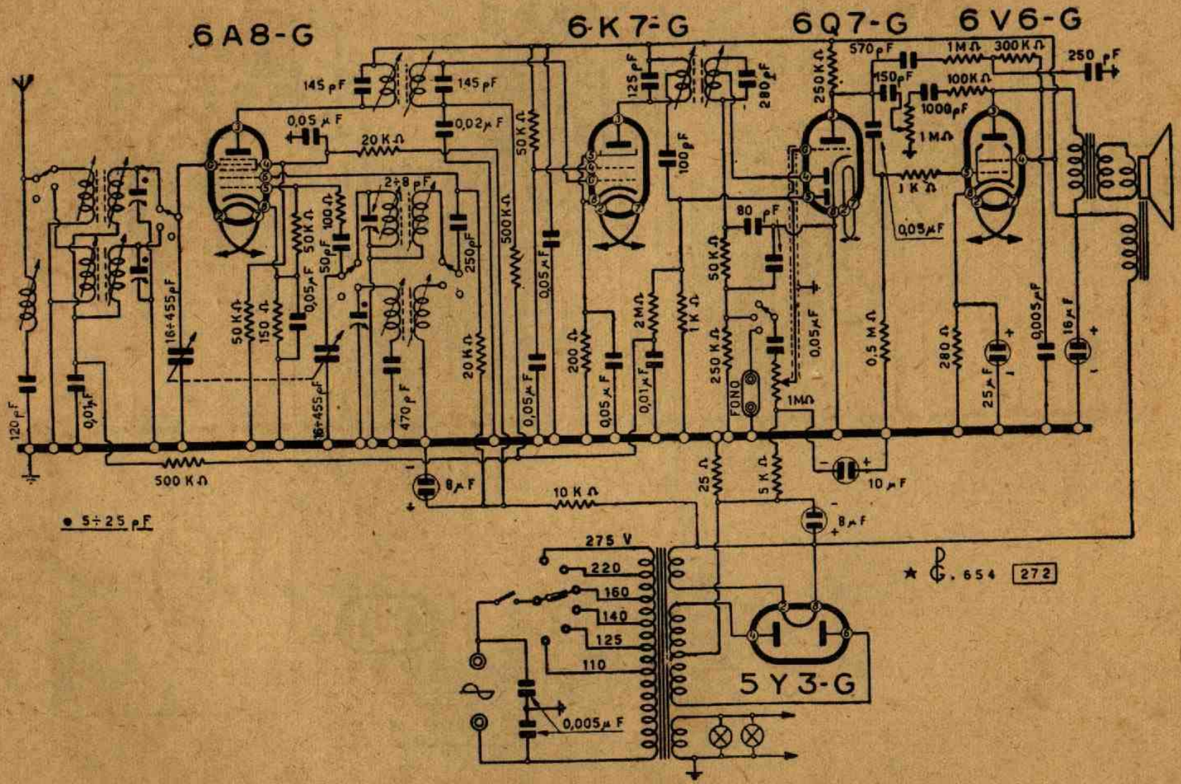
Lo schema elettrico del "C. G. E. 255 .."
